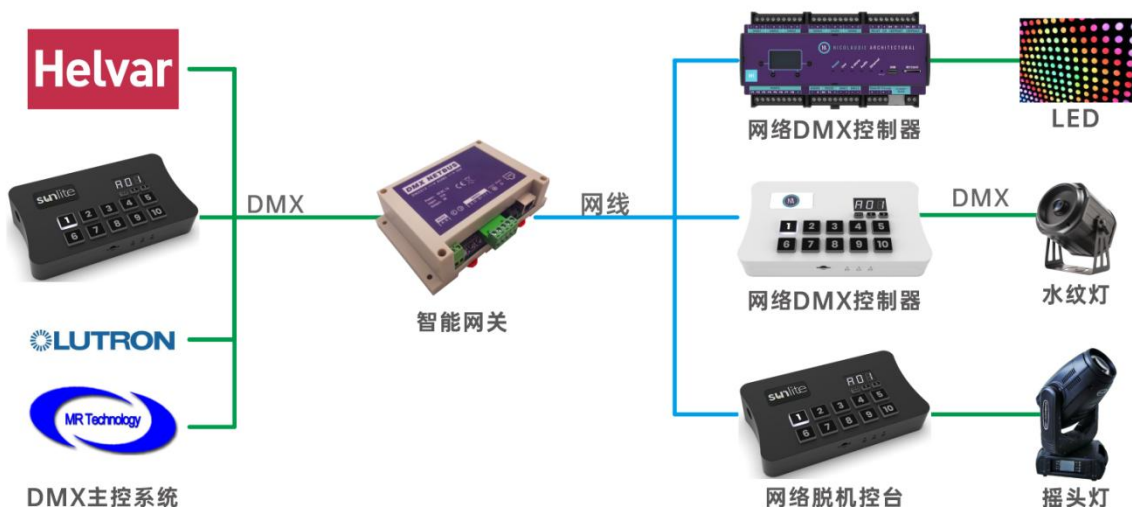
DMX 智能网系统图 (DMX系统联动)
