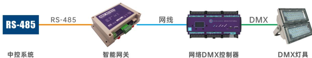
DMX 智能网关系统图 (RS485转换)
