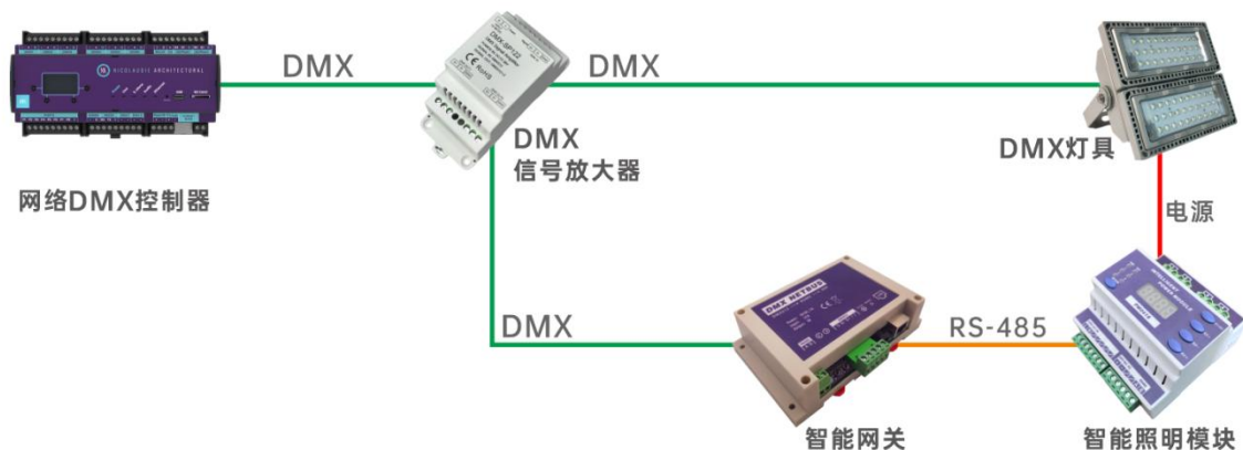
DMX 智能网系统图 (电源 & DMX 控制)
